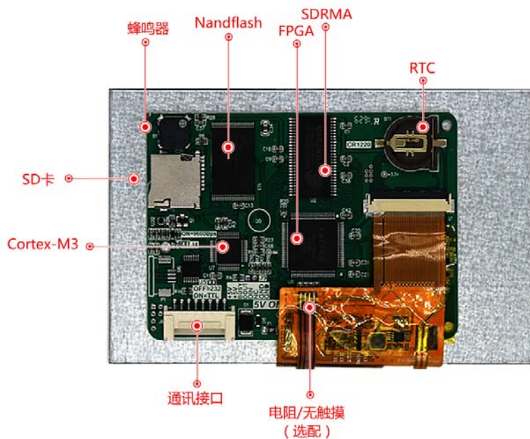
图 1-3 硬件配置图
