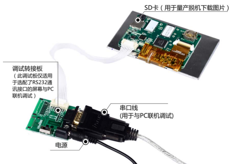
图 1-4 调试工具图
